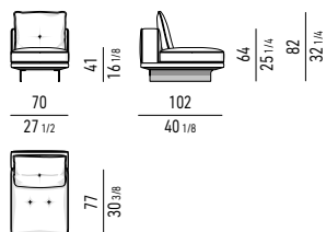
ELEMENTO CENTRALE CM 70 CENTRAL ELEMENT CM 70
